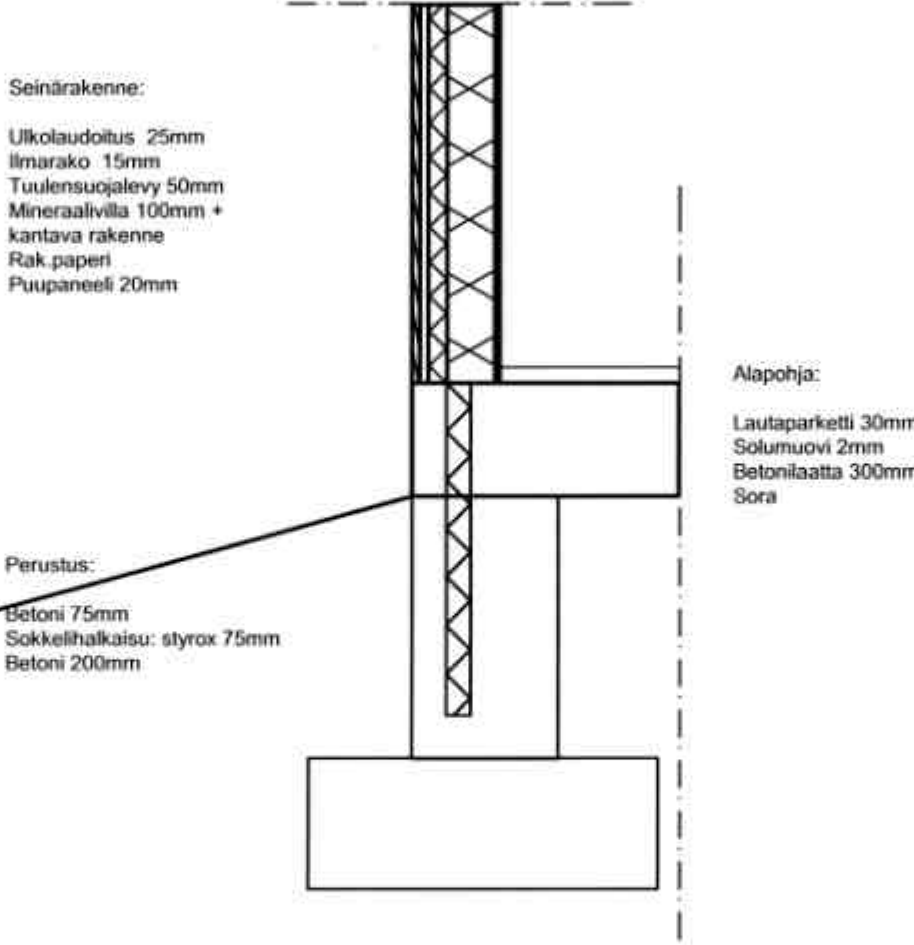
Rakenneleikkaus 1:20
