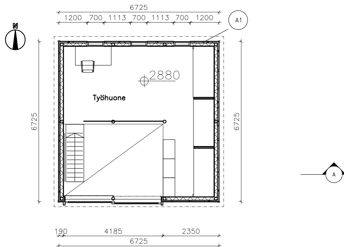
Pohjapiirros 2.kerros 1:100
