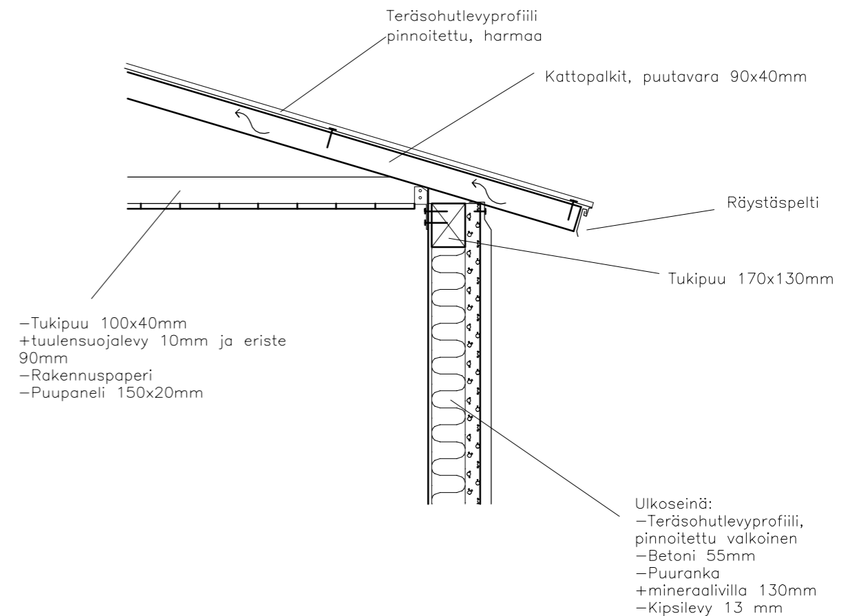
Det. A1 Rakenneleikkaus, räystä 1:20
