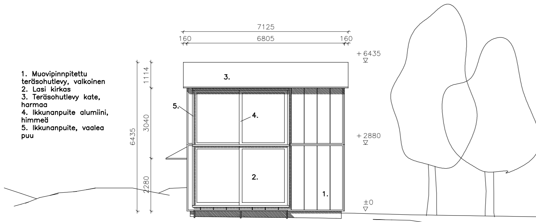
Julkisivuetaelästä 1:100
